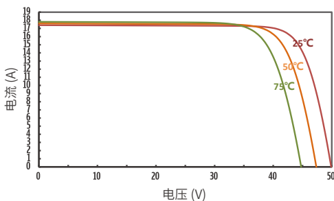
JT700SLk(B) 不同温度下的IV曲线
