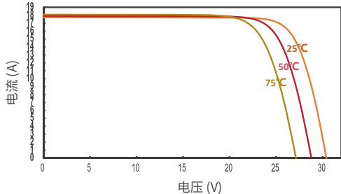
JT430SYk(B) 不同温度下的IV曲线
