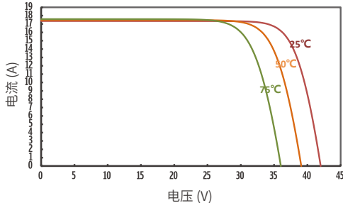
JT585SZk(B) 不同温度下的IV曲线
