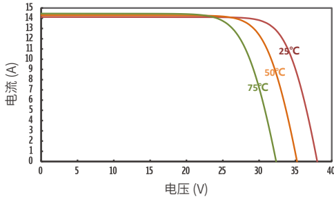
JT420SEt(L) 不同温度下的IV曲线
